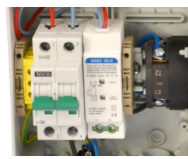
Automaat + automatische herinschakelbare differentieel (IDIL)
